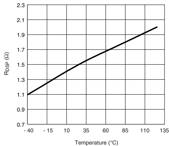
DH R_{DSP} vs. Temperature
