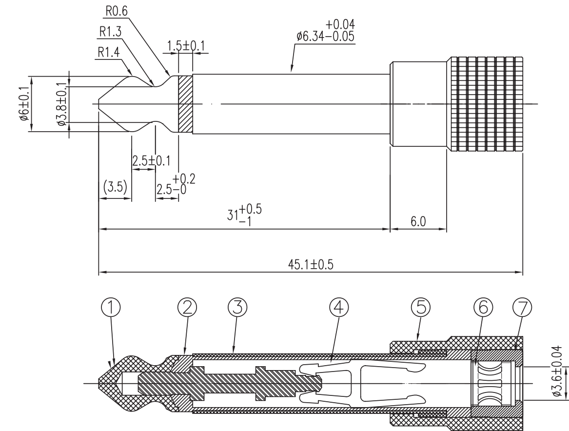
Ø6.3 Mono Plug
